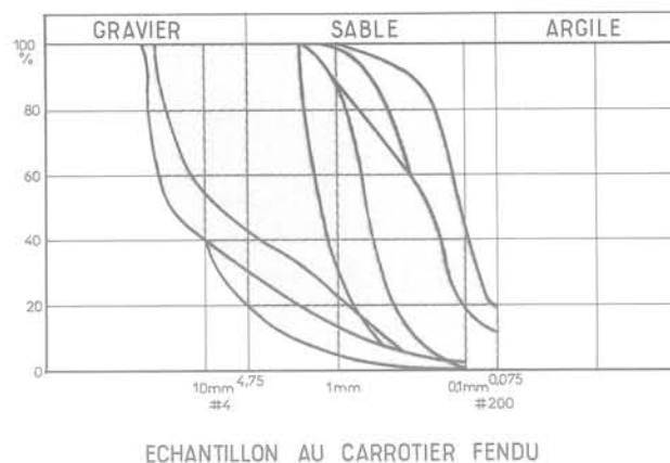
Fig. 6. — Exemples et fuseau des courbes granulométriques des alluvions à traiter.
